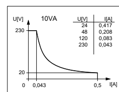
Leistungsdiagramm (maximale Werte)
