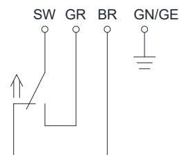
Anschlußschema (ohne Flüssigkeit)
