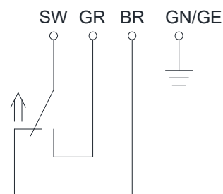
Anschlußschema (ohne Flüssigkeit)
