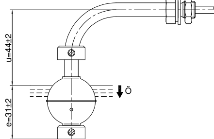
Anschlußschema Auslieferungszustand (ohne Flüssigkeit)
